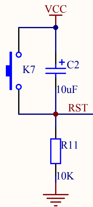
复位电路
