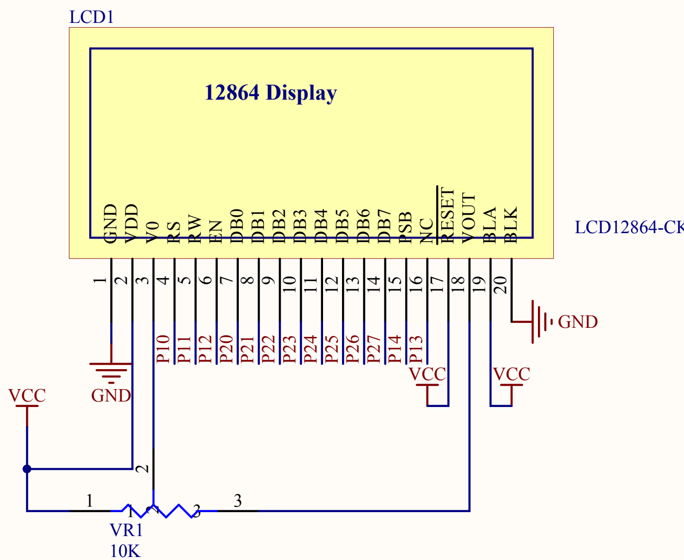
LCD12864 液晶显示
